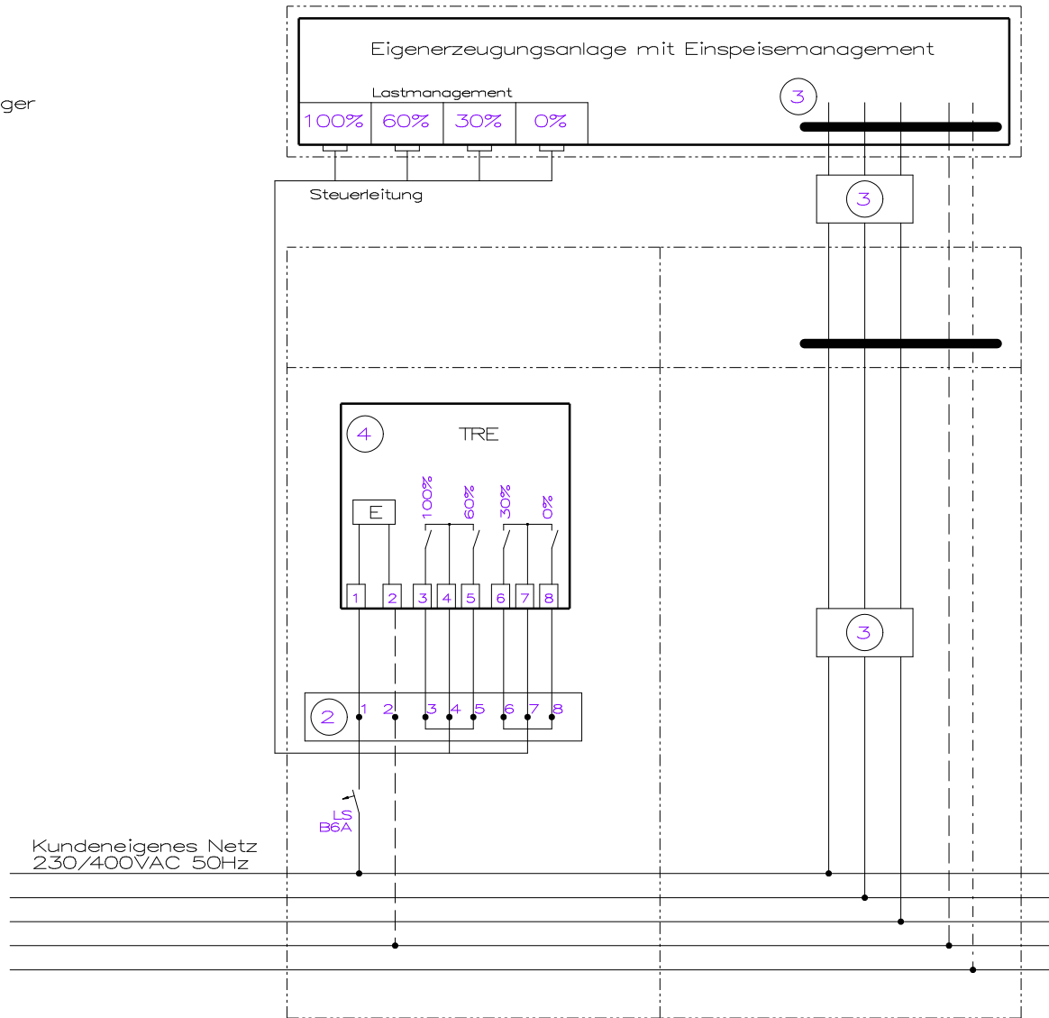
Verdrahtung und Installation mit Lastmanagementmodul bauseits
